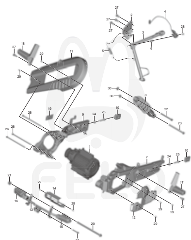
スイングアーム / リアサスペンション
