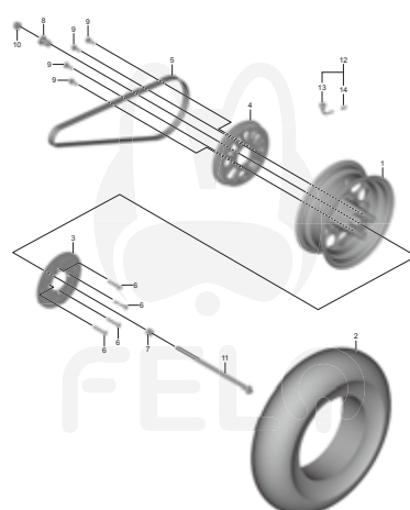
リアホイール
